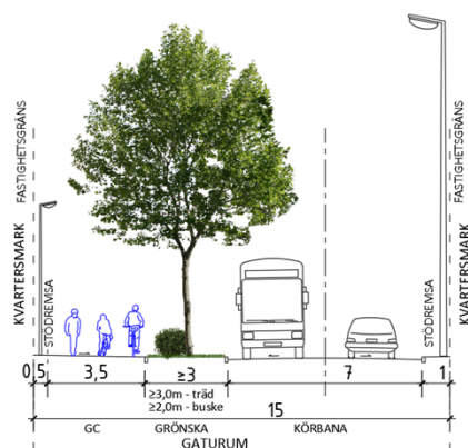
Figur 18. Principiell tvärsnitt av den centrala gatan (Gata 2). Total bredd min. 15 m inklusive stödremсор. Detta möjliggör 7,0 m körbana, min. 3,0 m grönremsa med trädplantering, 3,5 m GC-väg + stödremsa mellan 0,25 - 0,5 m samt stödremsa/vägren på ca 1 m.
