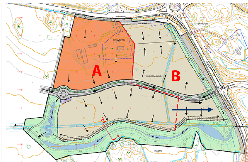
Figur 23. Koncept för avvattning inom planområdet enligt framtagen förprojektering och dagvattenutredning. Pilar visar åt vilket håll bör dagvatten rinna, röd streckad linje utgör gräns mellan västra (A) och östra (B) avrinningsområdet
