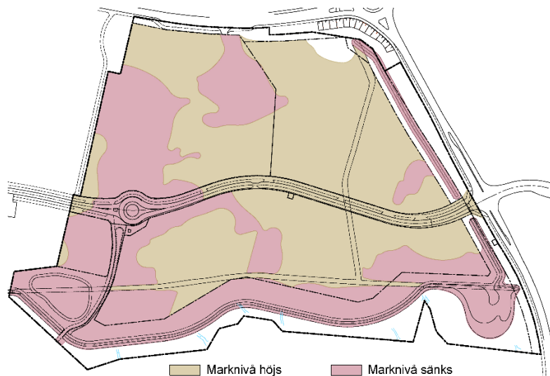
Figur 31. Ungefärlig justering av marknivåer enligt framtagen förprojektering.
