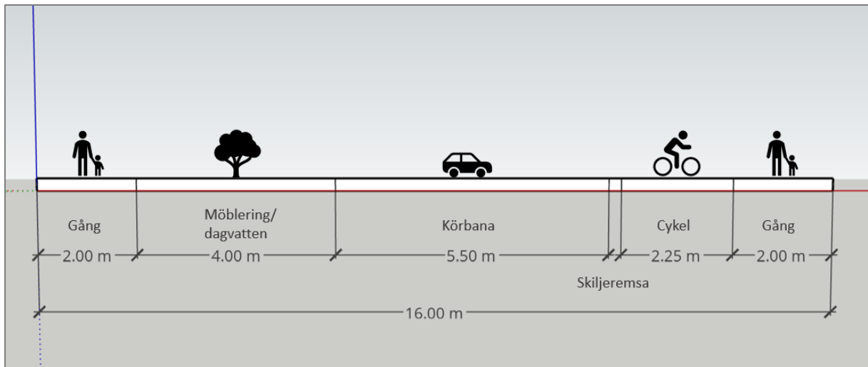
Figur 15. Förslag på gatusnitt, gatan mot skolan.
